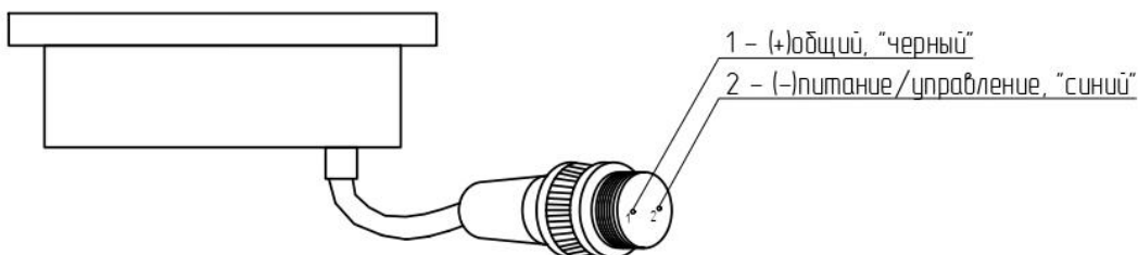
Схема подключения монохромного прожектора
