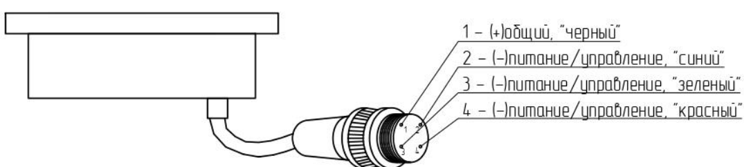
Схема подключения RGB-прожектора
