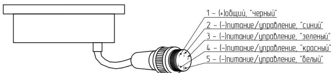
Схема подключения RGBW-прожектора
